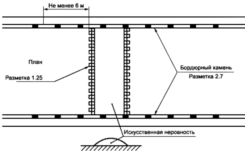
Рисунок 4 - Пример нанесения разметки 1.25 и 2.7 при устройстве ИИ
