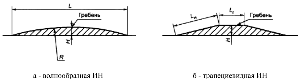
Рисунок 1 - Поперечные профили ИН
